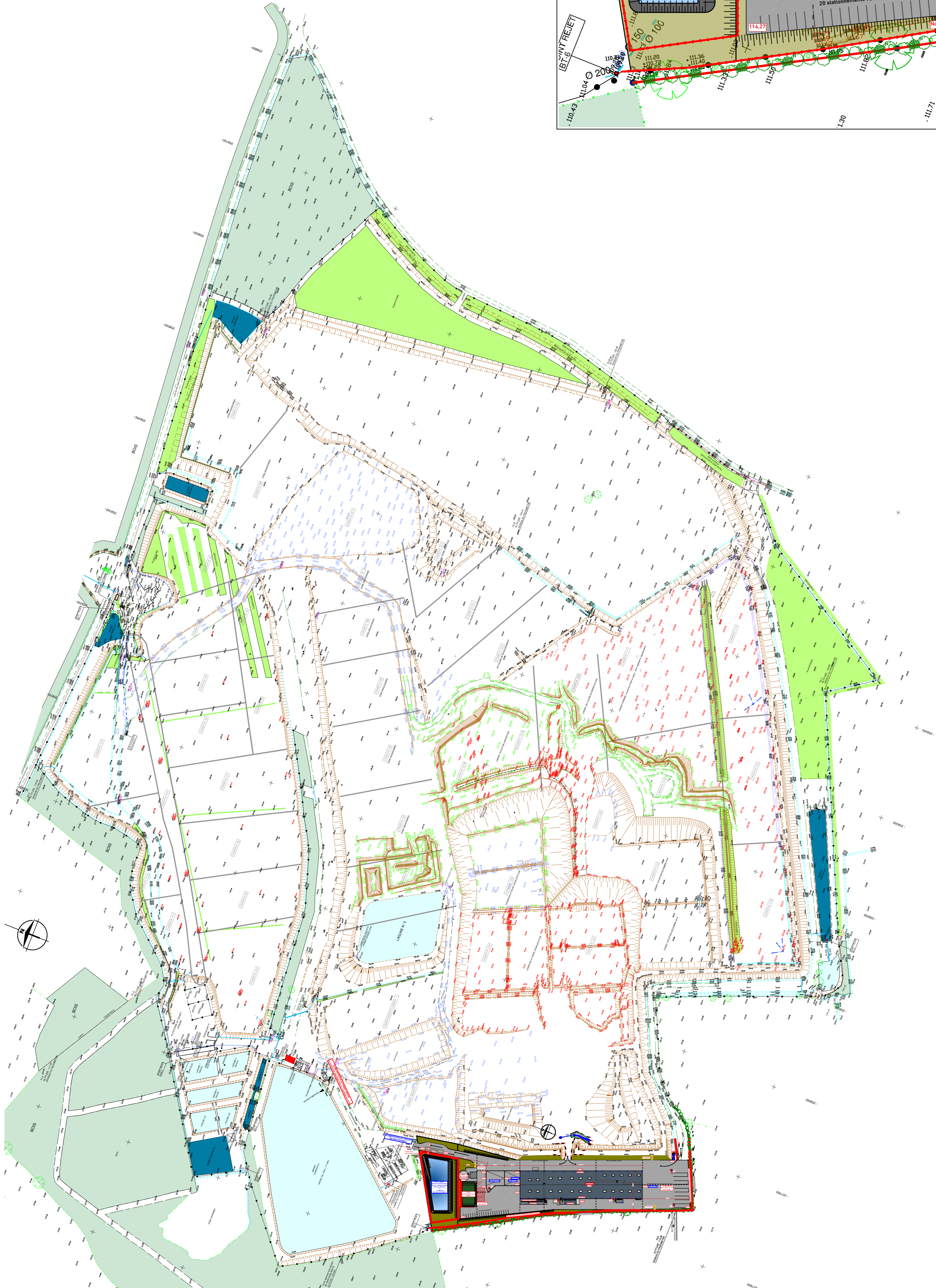
1:2000 Plan du site
